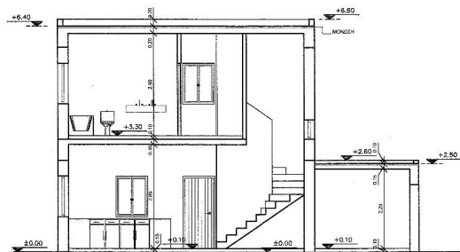
ΤΟΜΗ Α-Α
