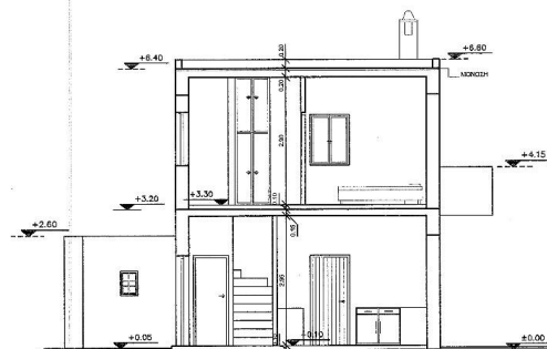
ΤΟΜΗ Β-Β
